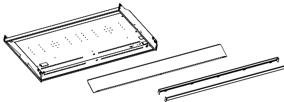
Luminaire Body
